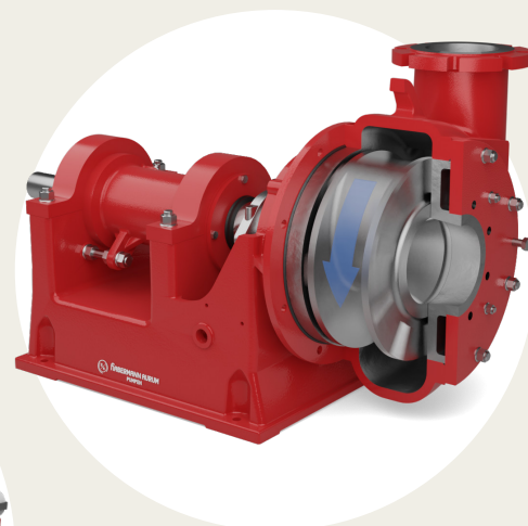
Baggerpumpe KBKM 150/400
