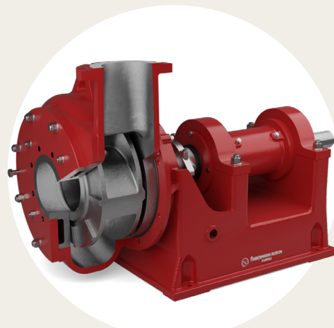
Baggerpumpe KBKM 150/300 mit freiem Wellenende
