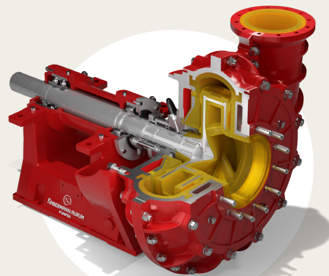
HPK mit Polyurethan APFlex® Auskleidung
