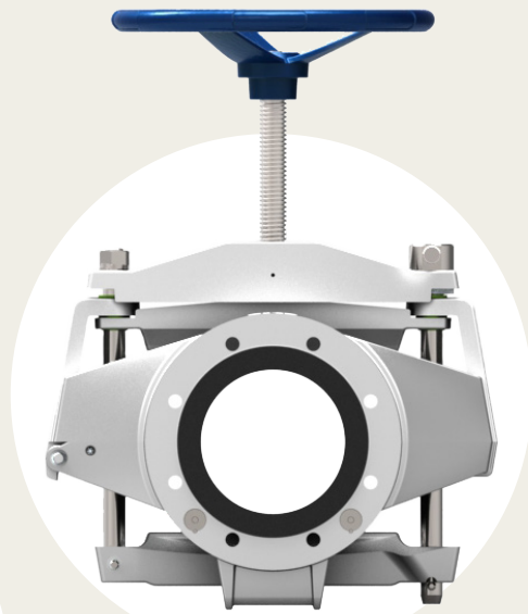
Quetschventil für stark abrasive Medien
