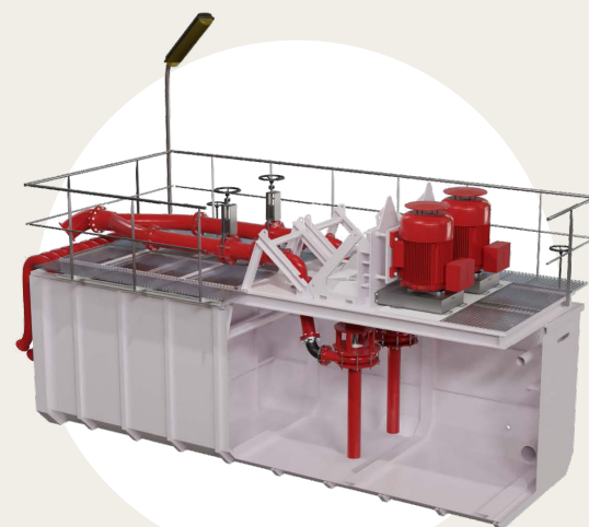
Baggerpumpe KBKM 150/400
