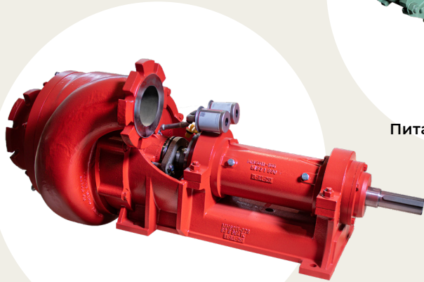
Насос для туннеля KB 100
