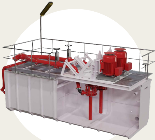
Дноуглубительный насос KBKM 150/400
