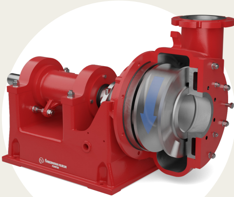
Дноуглубительный насос КВКМ 150/400
